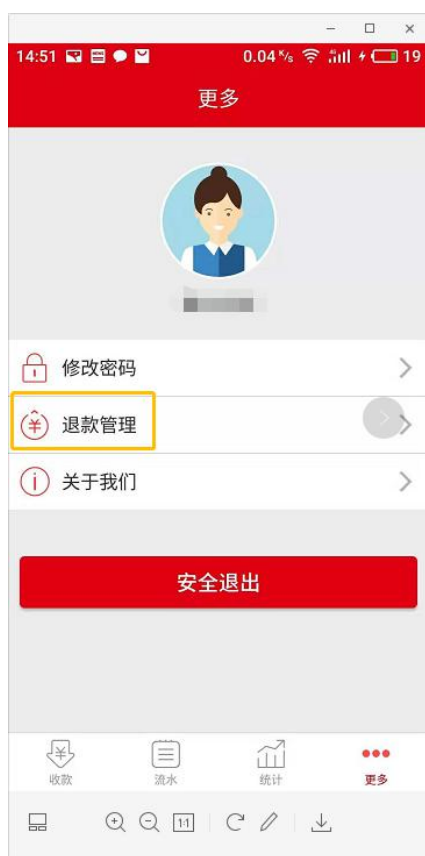
退款管理图3.6.2.1
